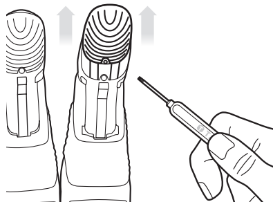
Entfernen der Fingerspitzen mit dem TASKA-Schraubenzieher
