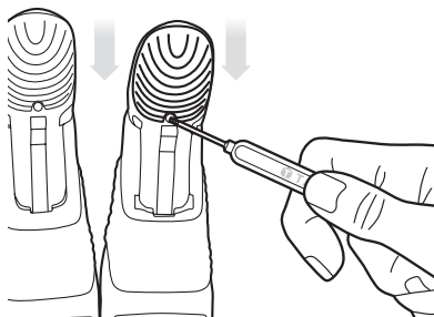
Positionieren und Anbringen einer neuen Fingerspitze
